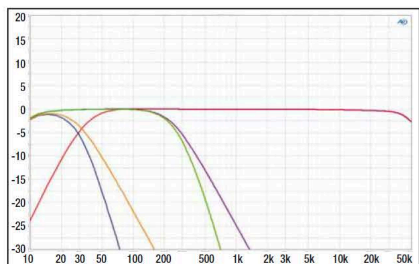
Die Stealth 1200.1 läuft ungefiltert geradeaus bis 50 kHz. Dert Tiefpass reicht bis 250 Hz und hat wahlweise 12 oder 24 dB/Okt. Flankensteilheit
