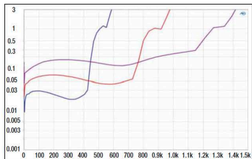
Die Stealth 1200.1 ist bärenstark mit bis zu 1250 Watt. Die Mehrleistung an niedriger Last wird mit steigenden Verzerrungen erkauft, die jedoch auch an 1 Ohm absolut ok sind
