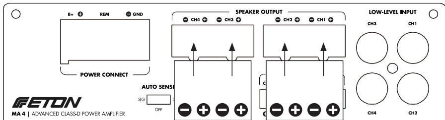
MA 4 Audio Ausgang MA 4 Audio output
