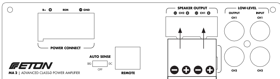
MA 2 Audio Ausgang MA 2 Audio output
