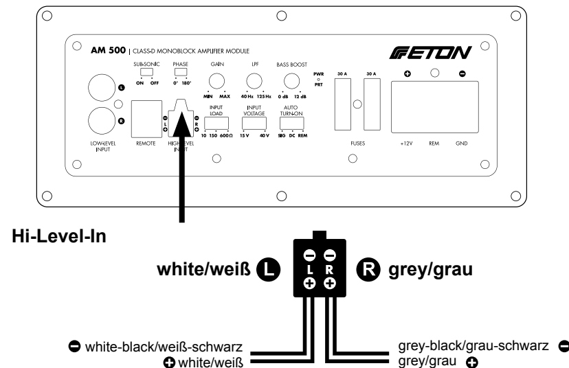
Anschlussdiagramm (High-Level)
