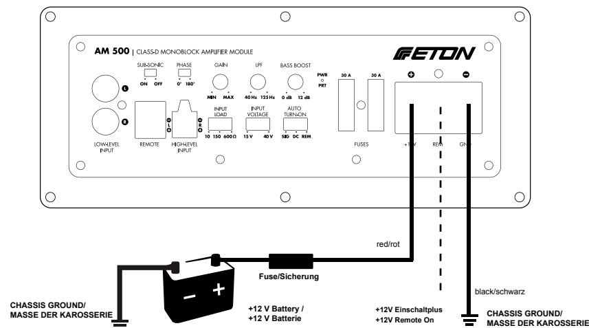
Anschlussdiagramm (Strom)
