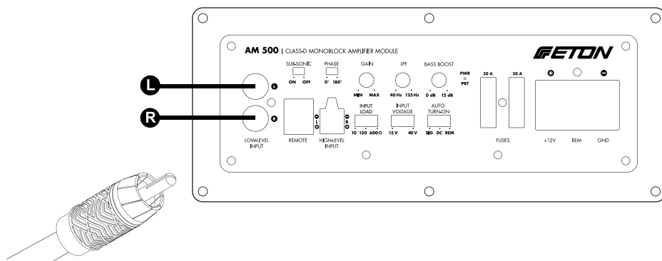
Anschlussdiagramm (Lo-Level / RCA Cinch)
